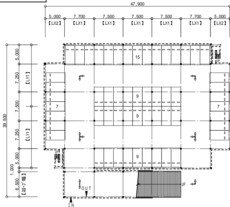
1階 平面図
